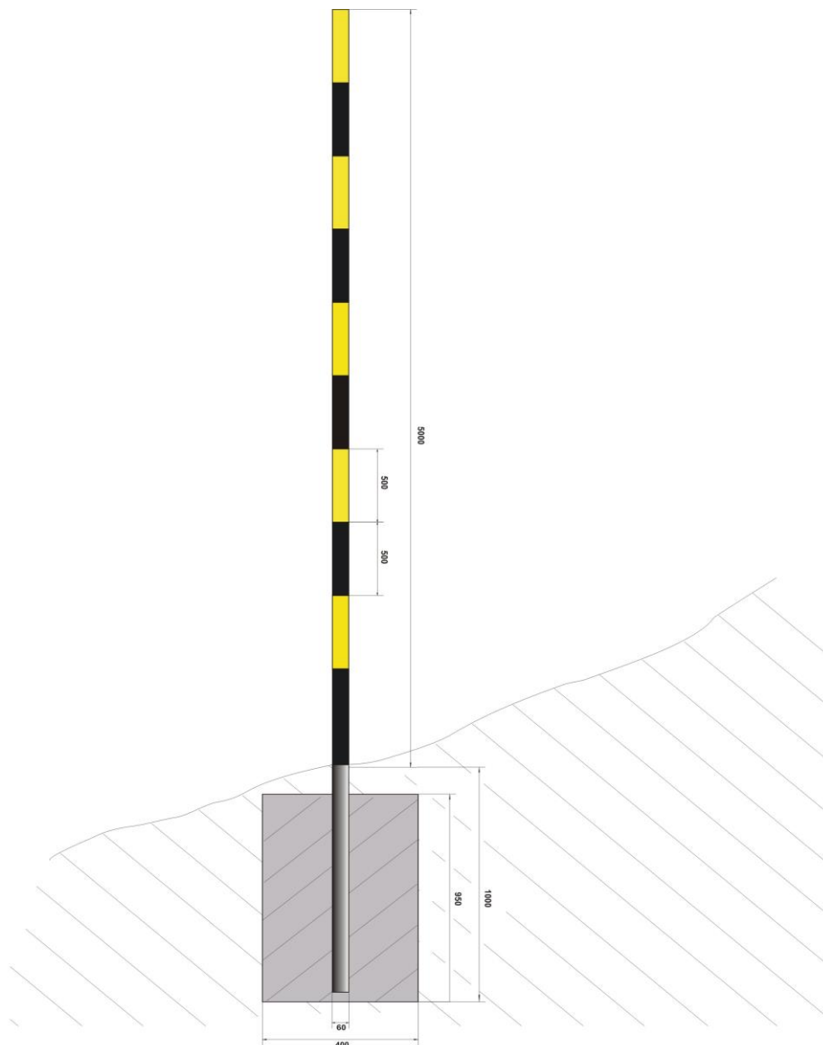
Фиг. 3 Поставяне на 6 м стълбове
