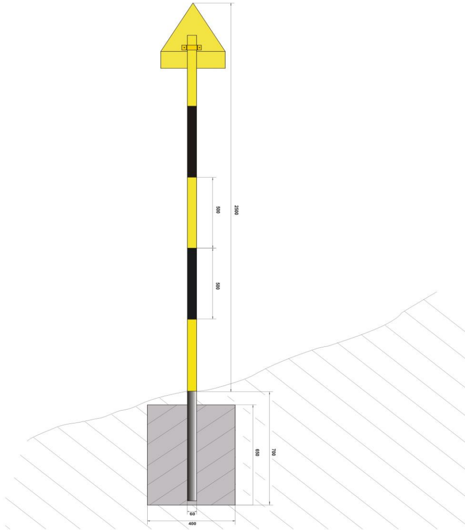
Фиг. 1 Поставяне на 3.2 м стълбове
