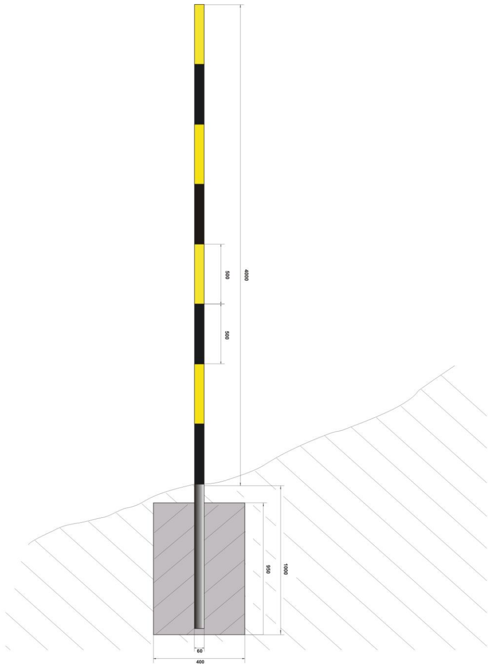
Фиг. 2 Поставяне на 5 м стълбове
